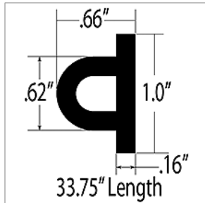
01377274 EXTRUSION, RUBBER, UPPER DOOR SEAL 36 DR AA
