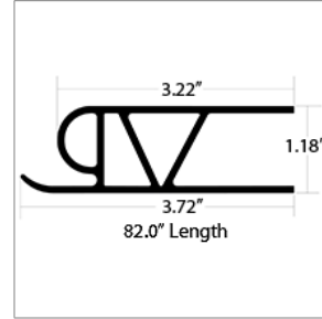
01380708 RUBBER,DOOR NOSING,FLUSH JACKKNIFE DOOR
