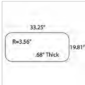
01565126 GLASS,CLEAR,STORM,UPPER,REAR EM DOOR
