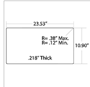
01773134 GLASS,UPPER,O/O ENT DR LAM CLR CV
