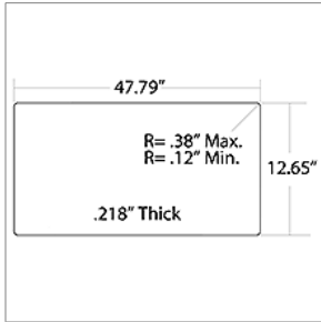
01781285 GLASS, LWR, O/O ENT DR, LAM CLR, 24.75 TC
