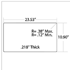
01773142 GLASS,UPPER,O/O ENT DR TEMP CLR CV
