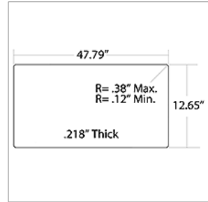
01781293 GLASS, LWR, O/O ENT DR, TEMP CLR, 24.75 TC
