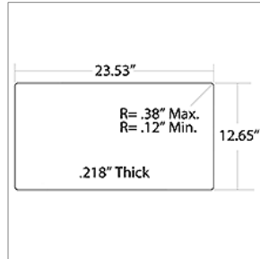
01773092 GLASS,UPPER,O/O ENT DR LAM 70 LT GRD TC
