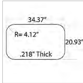
01110048 GLASS,RED,UPPER,TEMPERED
