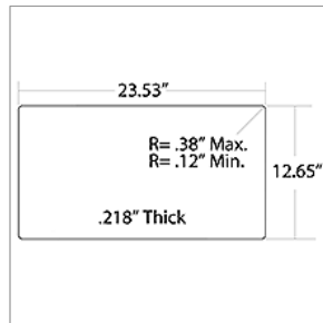
01773084 GLASS,UPPER,O/O ENT DR TEMP CLR TC
