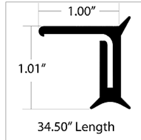
01695915 EXTRUSION, RUBBER, UPPER ENT DOOR SEAL, 34.50
