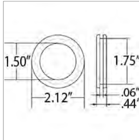
00421792 GROMMET,1 3/4 X 1/16 X 1 1/2
