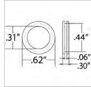
02003168 GROMMET, RUBBER,
