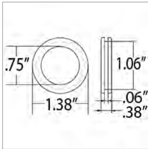
02003192 GROMMET, RUBBER, FC
