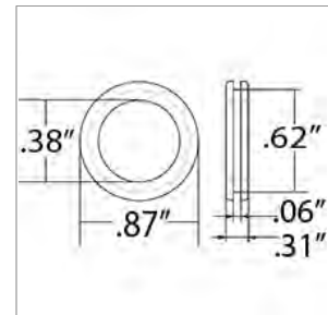
02003218 GROMMET, RUBBER, 3/8 ID
