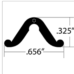
01233964 TRIM,VINYL,GRILLE BAR,FILLER
