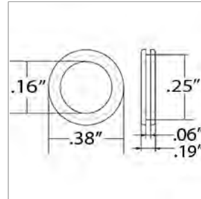
02003150 GROMMET,CHASSIS,COWL WIRING
