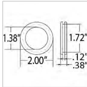
01610450 GROMMET, RUBBER, 1.38 ID X 1.718 OD
