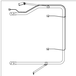
00127505 ARM ASSY,MIRROR,PASSENGER,OPEN VIEW,ROSCO
